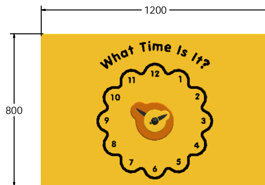
FICLOCK3 FICLOCK3-AL-WP
